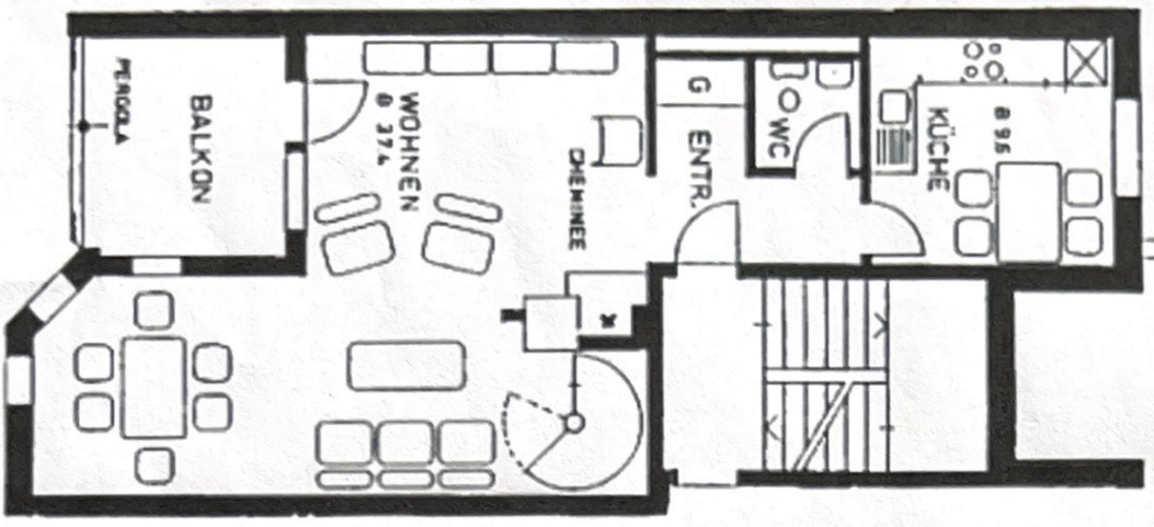
1. Obergeschoss
