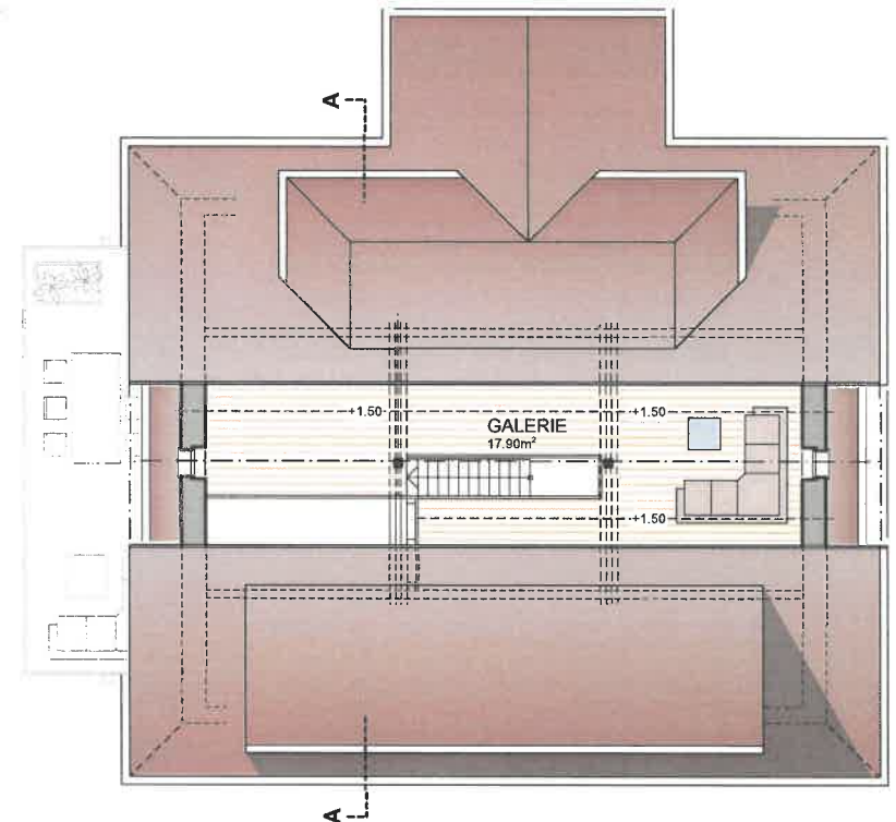
OBERGESCHOSS 1:100
