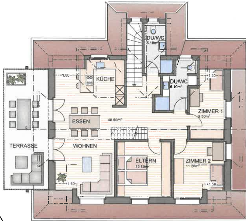
DACHGESCHOSS 1:100
