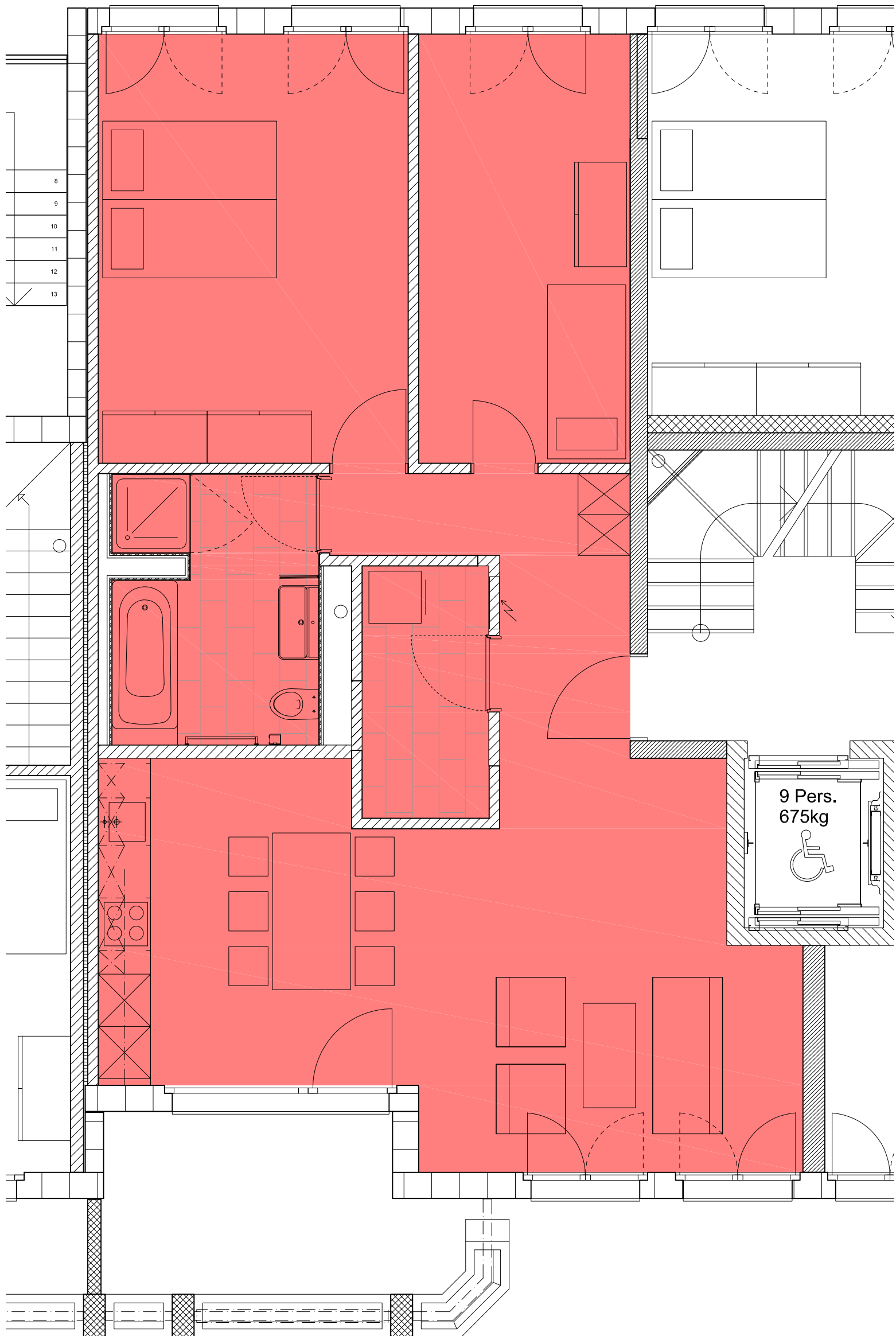
Haus 277 1.Obergeschoss Wohnung 277c-102
