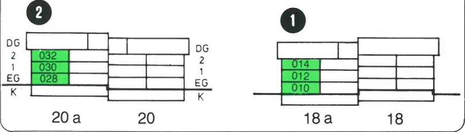
QUERSCHNITT - SCHEMA
