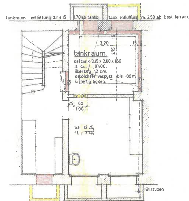
grundriss untergeschoss.
